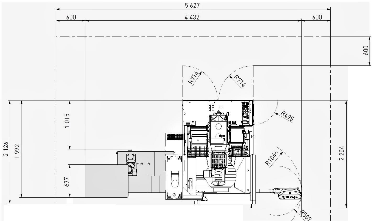
Вид сверху
