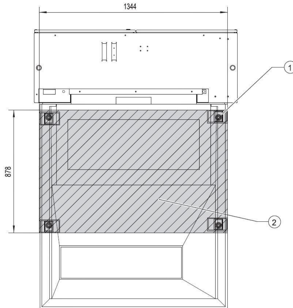
План фундамента
