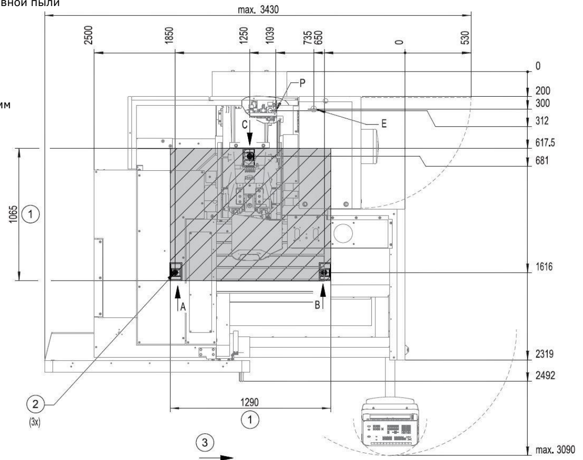
План фундамента
