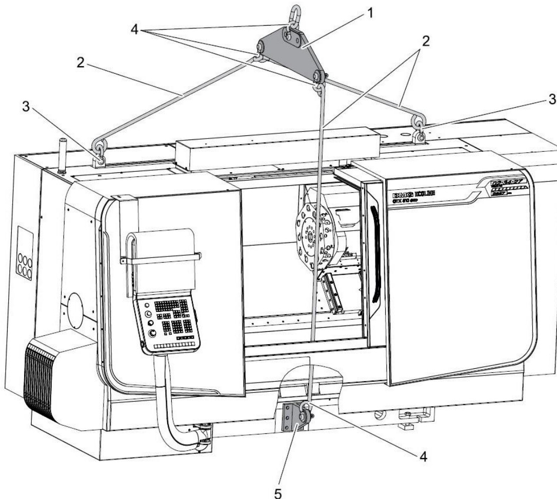
СХЕМА СТРОПОВКИ СТАНКА СТХ 510 ecoline
