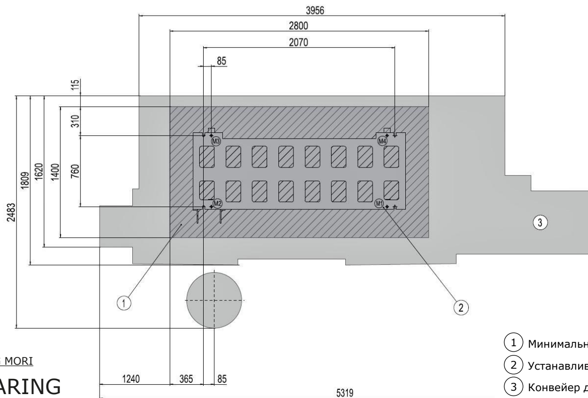
План фундамента
