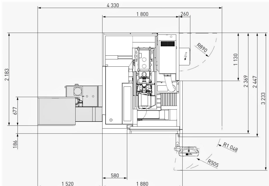
Вид сверху
