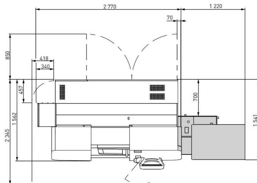
Вид сверху
